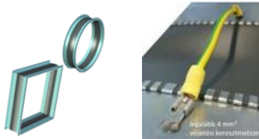
F-1. ábra: légszatórnába építendő hőtágulási kompenzátorok; potenciálkiegyenlítés
